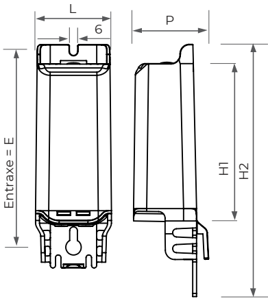
DL-Pak 70/100/200
