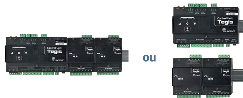
Unité de contrôle + 2 modules de surveillance (29 entrées de surveillance TOR au total)
